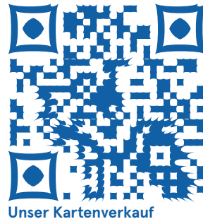
Unser Kartenverkauf
